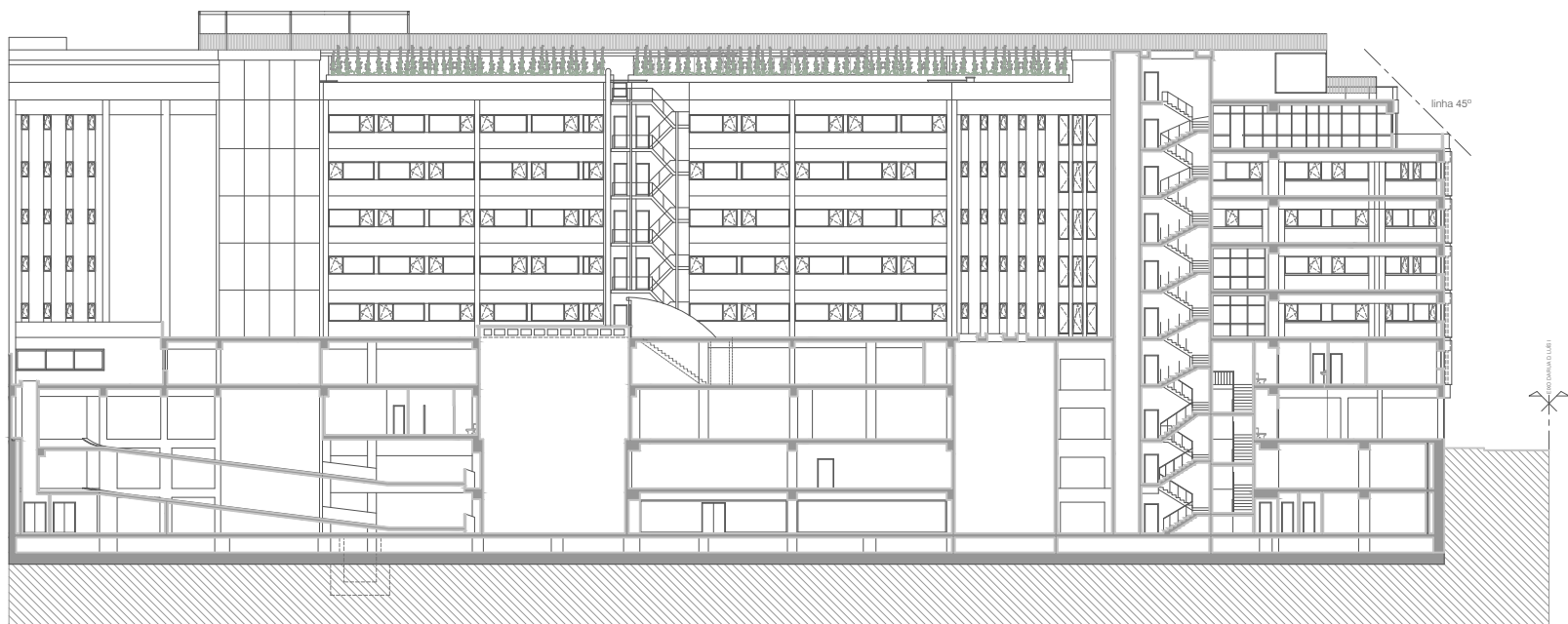
ALÇADO/CORTE POSTERIOR
